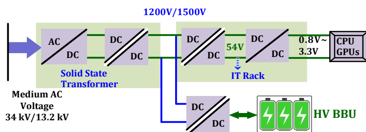
圖 1 未來 AI 伺服器系統之供電架構
